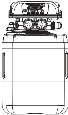
a) Enthärtergehäuse (einschließlich Druckbehälter mit Medienfüllung, Clack-DV-Regelventil)
